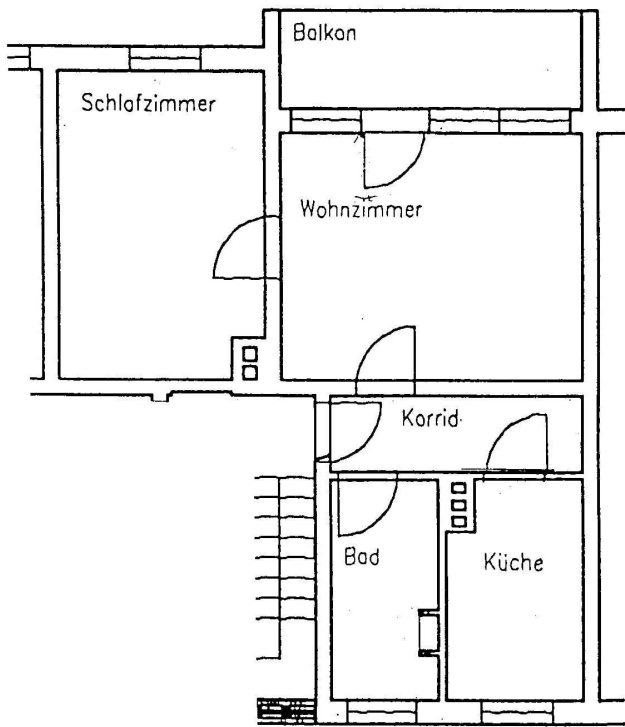
Grundriss
