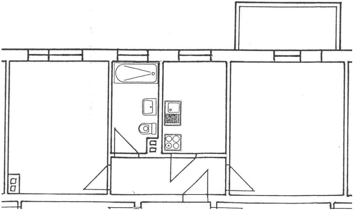
Grundriss
