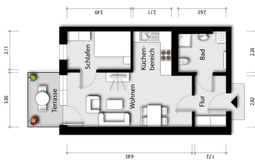
Grundriss (Möbel nur Einrichtungsbeispiel, WE wird ohne Möbel vermietet)
