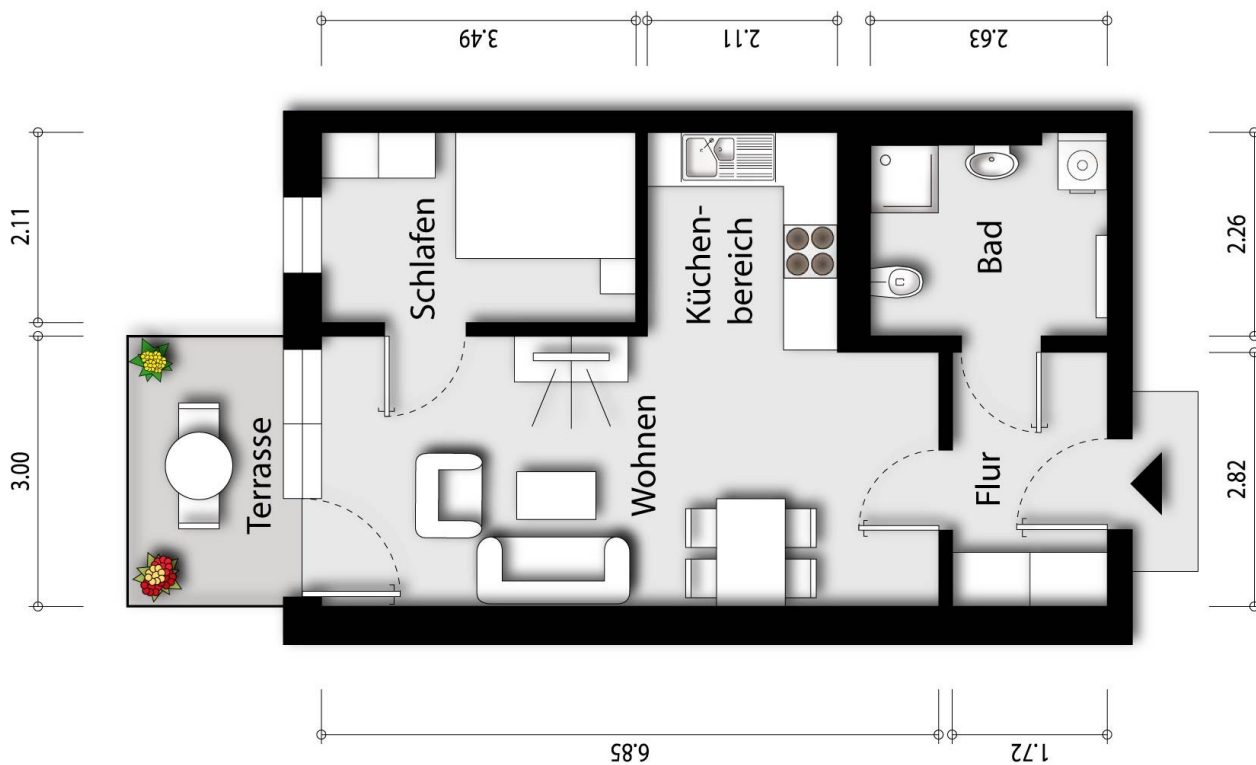
Grundriss (Möbel nur Einrichtungsbeispiel, WE wird ohne Möbel vermietet)
