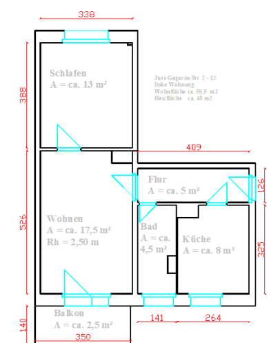
Grundriss
