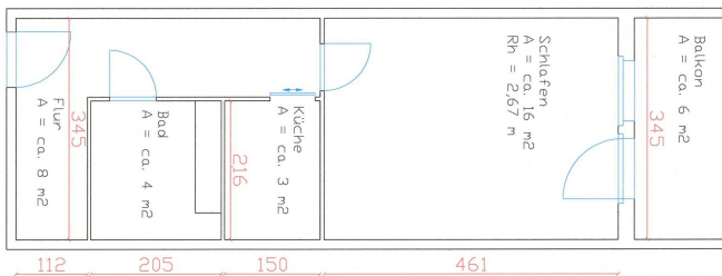
Grundriss
