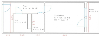
Grundriss
